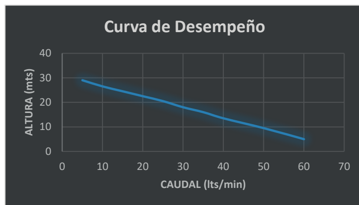
Cuadro de prestaciones PKm60-MD
