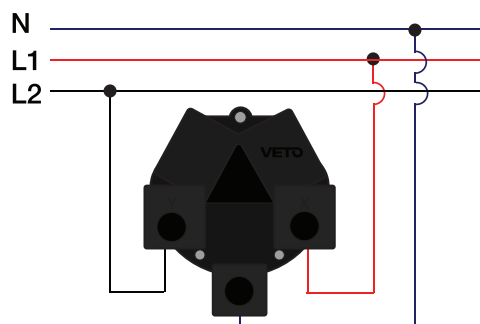
Diagrama de Instalación Toma Nema 10-50A
