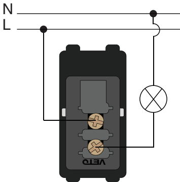
Diagrama de Instalación Interruptores
