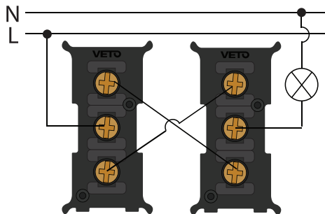
Diagrama de Instalación Conmutadores
