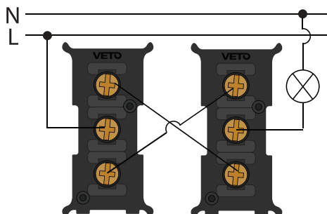
Diagrama de Instalación Conmutadores
