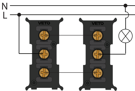
Diagrama de instalación
