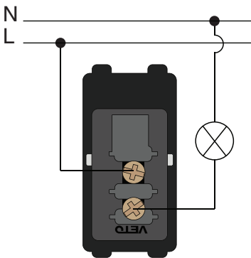
Diagrama de instalación Interruptores
