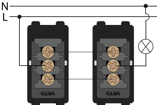
Diagrama de Instalación Conmutadores
